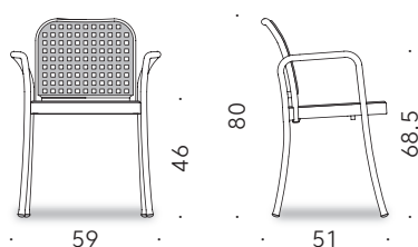
Silla apilable con brazos.
