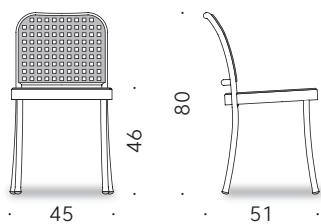
Sedia senza braccioli.
