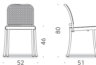
Chaise empilable sans accoudoirs.
