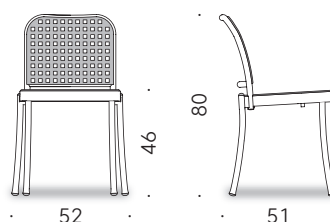
Stapelstuhl ohne Armlehnen.
