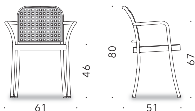
Stuhl mit Armlehnen.
