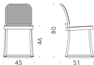
Stuhl ohne Armlehnen.
